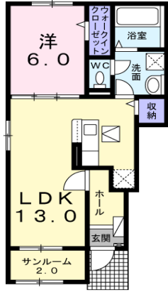
間取図
